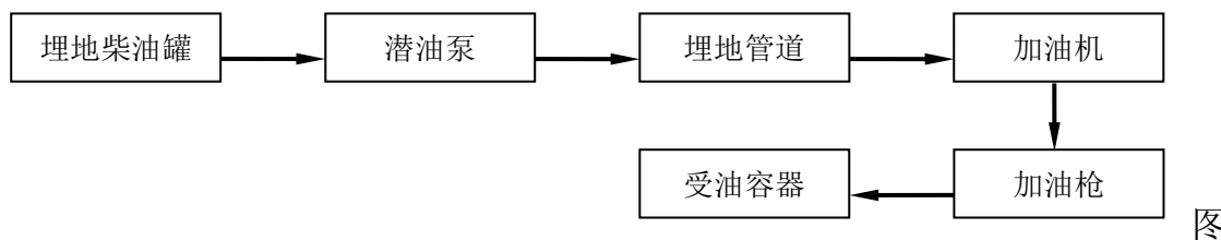
2.3-4 柴油加油工艺流程图示意简图
